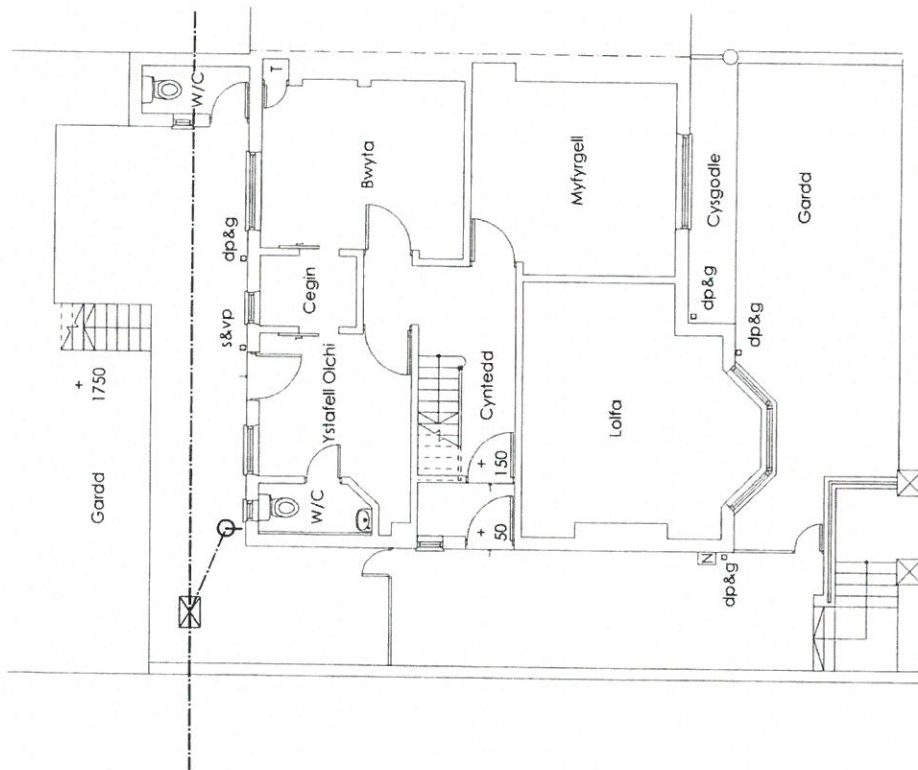
Llawr Gwaelod
