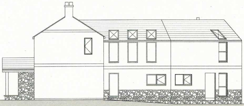
RHS Elevation
