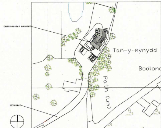
Block Plan 1 : 500
