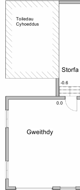
2 Cynllun Llwr Arfaethedig 1 : 100
