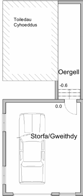
1 Cynllun Llwr Presennol 1 : 100
